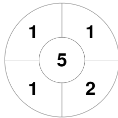
HAR
